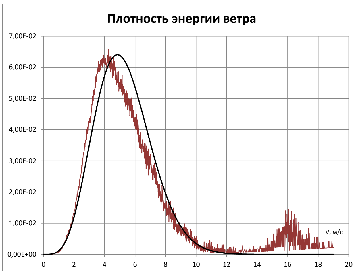
Рис.2 Плотность энергии скоростей ветра и соответствующей плотности энергии ветра. (РБ, Минский р-н, высота измерений 15 м, отметка над уровнем моря 265м, среднее значение P_{ср}=29,3 \text{ Вт/м}^2 , что соответствует среднекубической скорости V_{срк}=3.67 \text{ м/с} , P_{ср}=r_0/2 * V_{срк}^3 = 1,185/2 * 3,67^3 = .29,3 \text{ Вт/м}^2 )
